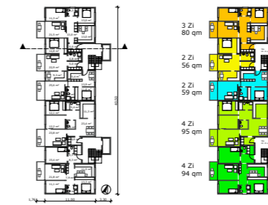
Grundrisse (N2) 1.-8.OG M1:200
