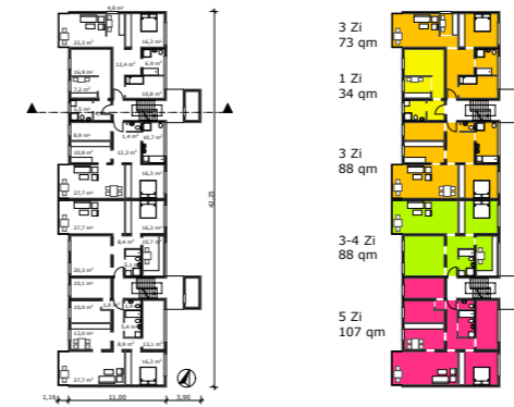
Grundrisse (B) 1.-8.OG M1:200
